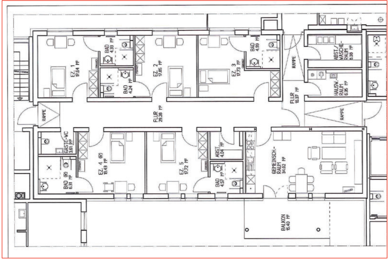
1. Obergeschoss
