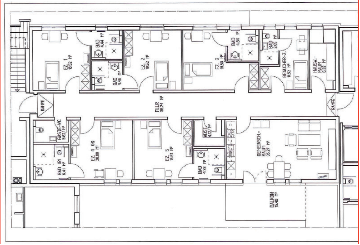
2. Obergeschoss
